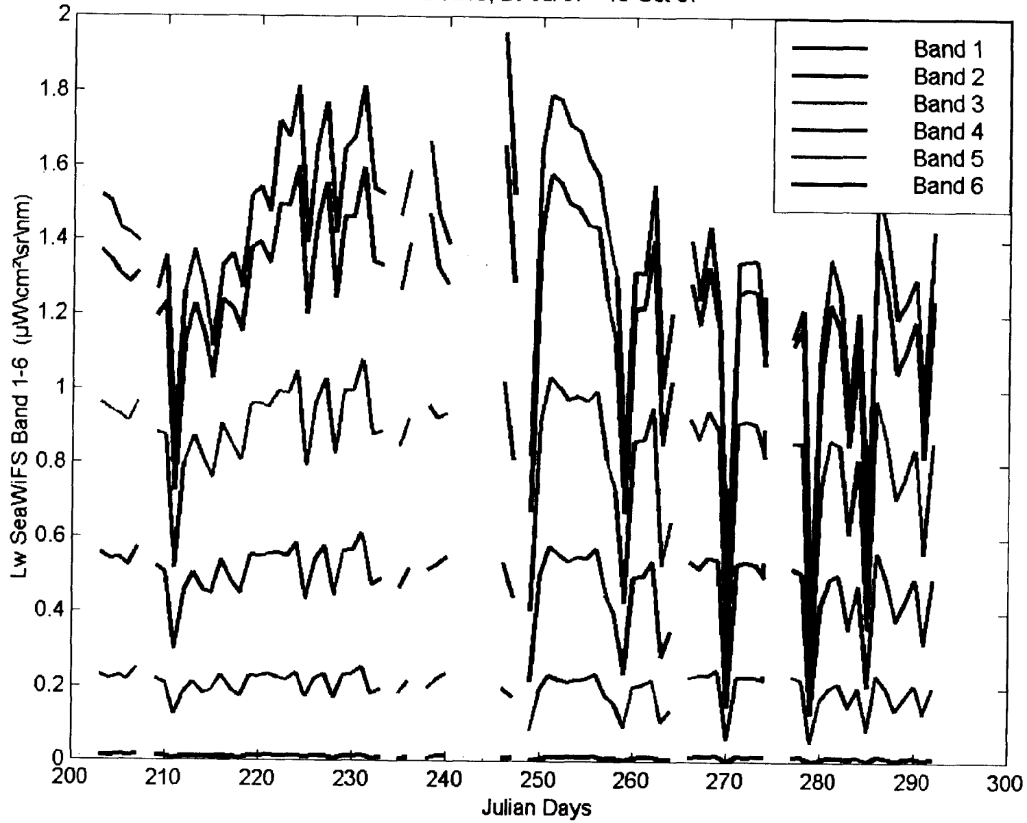
MOBY203, 20 Jul 97 - 19 Oct 97
